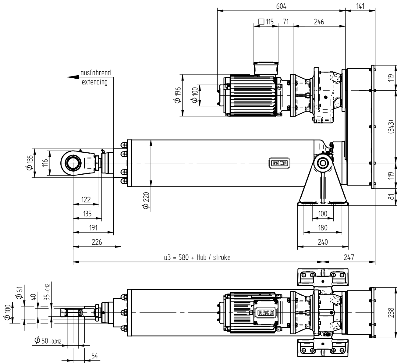
RACO-Elektrozylinder® Baugröße 8 Bauform N RACO Electric Actuator Size 8 Type N
